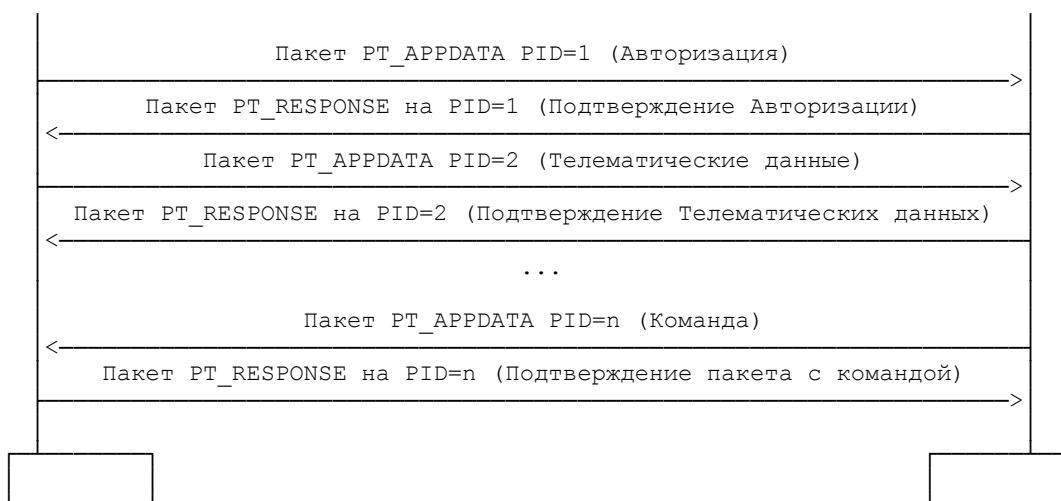
Рисунок N 3. Взаимодействие абонентского терминала и аппаратно-программного комплекса на уровне пакетов Транспортного уровня
